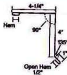
Snap-Lok Rake
