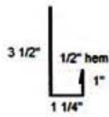
J - trim
